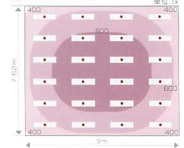
照度シミュレーション
