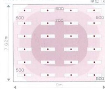
照度シミュレーション
